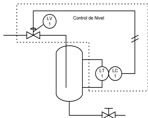
Figura 3. Esquema del sistema de llenado del depósito
